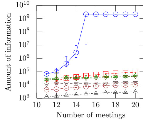
(d) Information complexity
