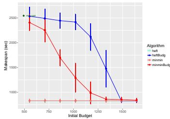
(d) Cyber, 90 tasks, \sigma = 0.50
