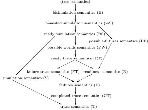
Fig. 1. The ltbt-spectrum
