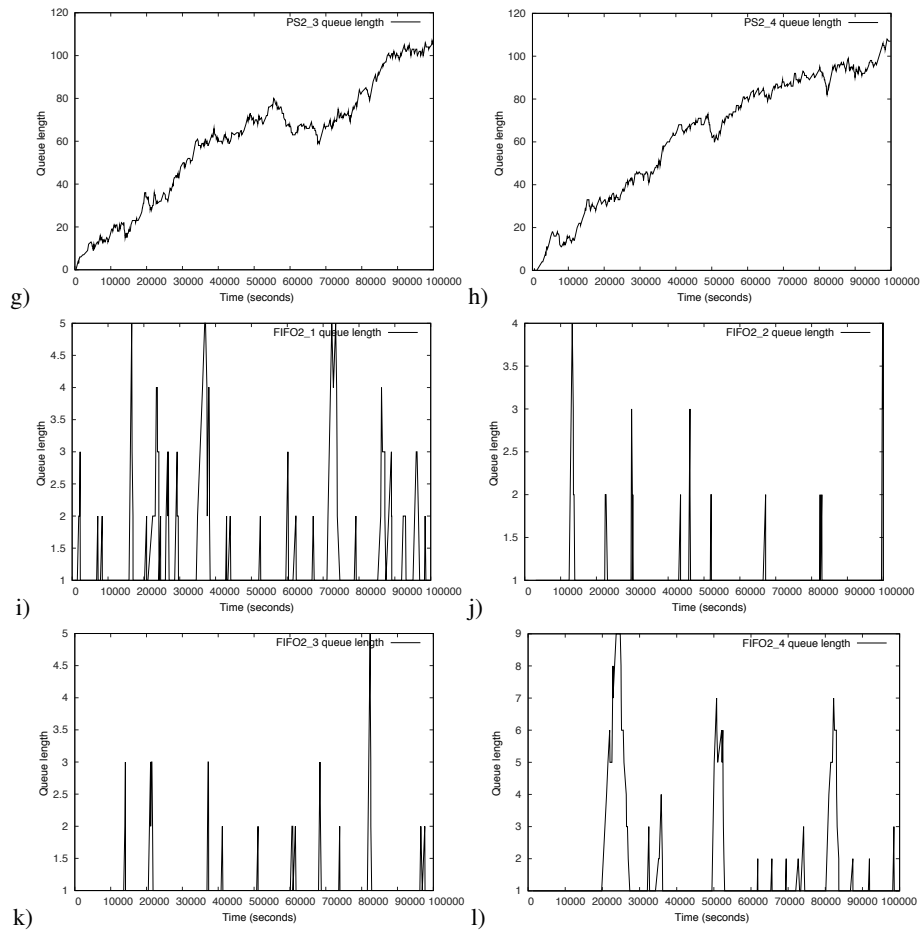
Fig. 10. Sample queue length history for case IV with 500[\text{requests}/\text{s}] : g) PS2_3, h) PS2_4, i) FIFO2_1, j) FIFO2_2, k) FIFO2_3, l) FIFO2_4.
