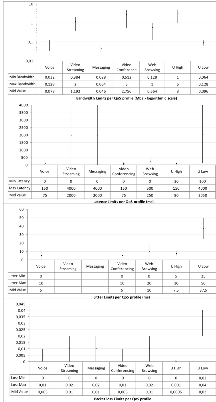
Fig. 3. QoS Profiles
