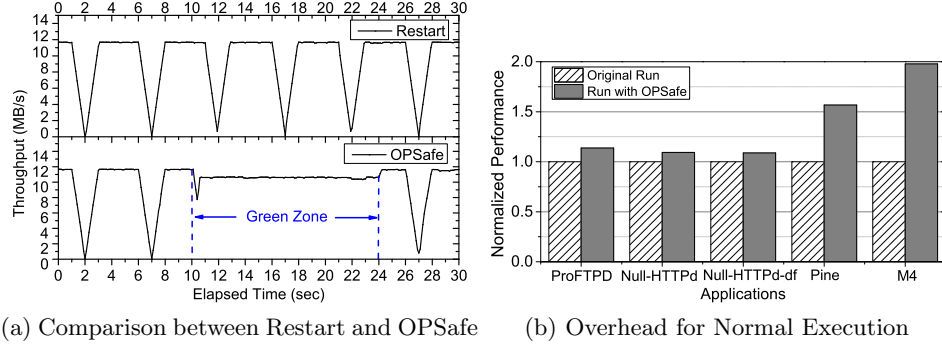
Fig. 2. OPSafe Evaluation
