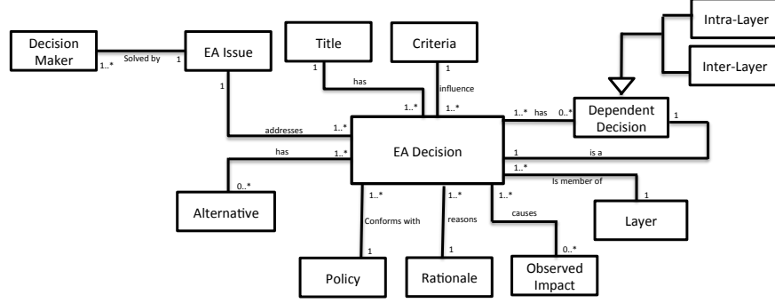
Fig. 1. The EA Anamnesis meta-model
