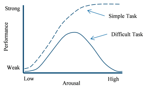
Fig. 1. Yerkes-Dodson law [13]
