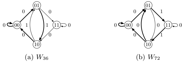
Fig. 5: De Bruijn graphs for W_{36} and W_{72}
