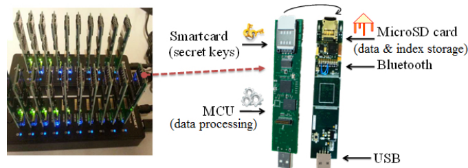
FIGURE 5 – Sondes sécurisées (SP)
