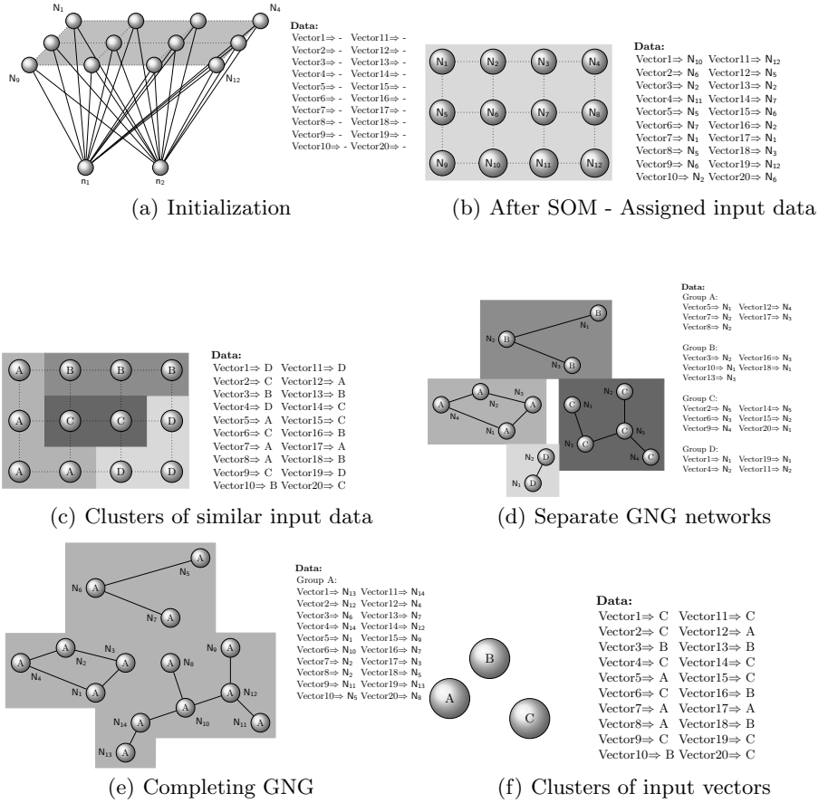
Fig. 1. Combination of SOM and GNG
