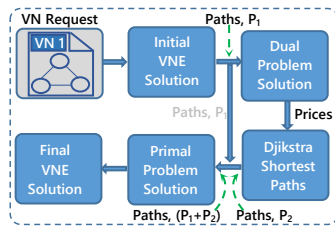
Fig. 1. PaGe-VNE
