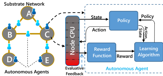
Fig. 2. RL-DRA
