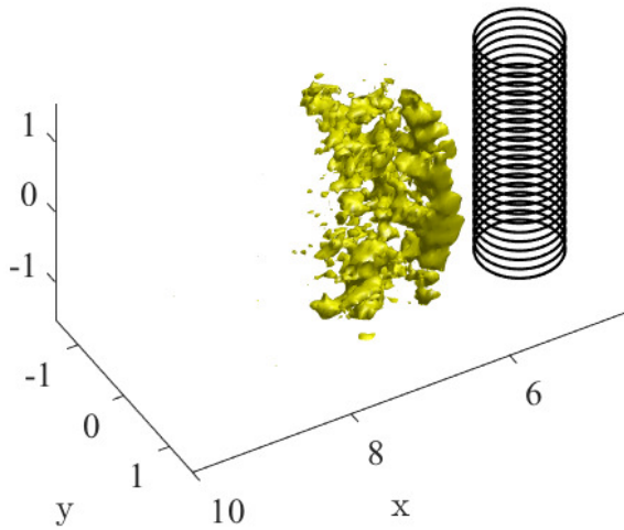
(d) \sqrt{\lambda_3}tr(\mathbf{z}_3) = 0.007
