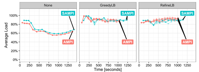
(d) Average Load and makespan using the Ligurian workload.
