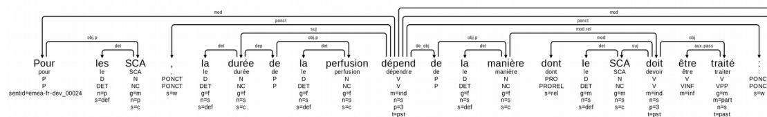
Figure 1: Dependency parse for the sentence “For the ACS [Acute Coronary Syndromes], the duration of the IV depends on the way the ACS should be treated: it can last a maximum of 72 hours for patients who need to take drugs” [In the original French: “Pour les SCA, la durée de la perfusion dépend de la manière dont le SCA doit être traité: elle peut durer jusqu’à 72 heures au maximum chez les patients devant recevoir des médicaments.”]
