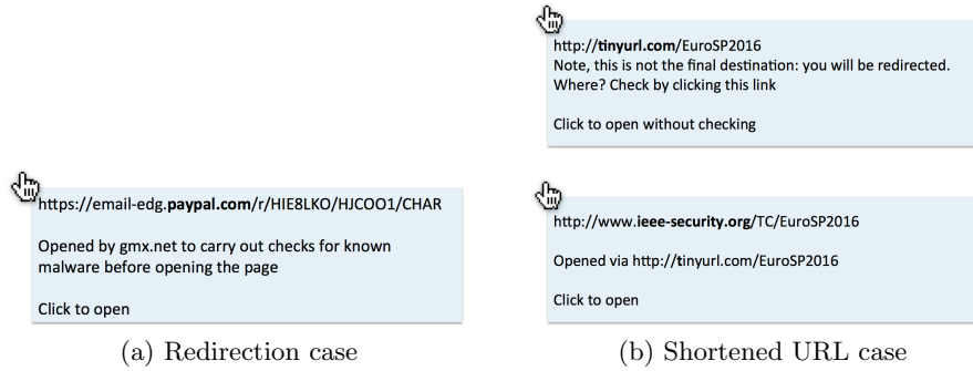
Fig. 3: Example tooltips
