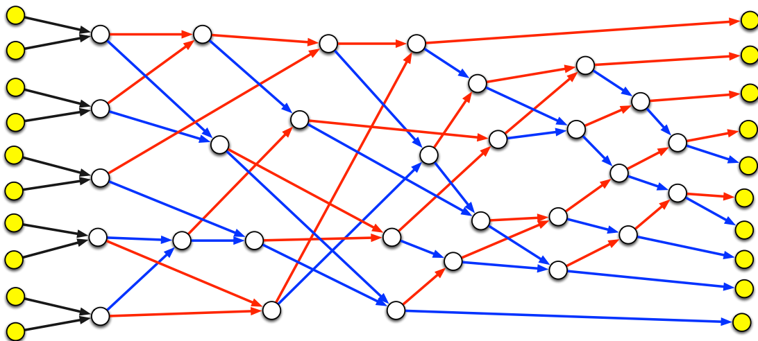
Graphe orienté pour trier dix nombres.
