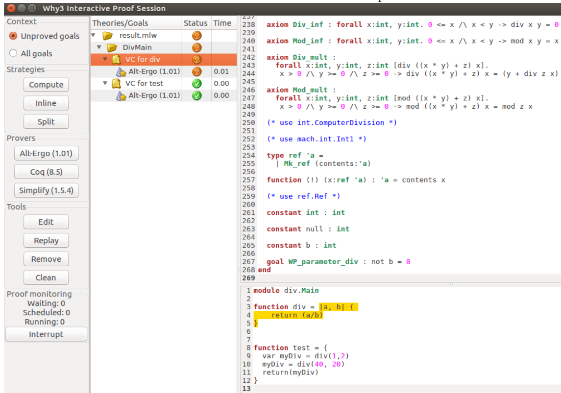
FIGURE 5 – Preuve de la fonction div sans spécification
