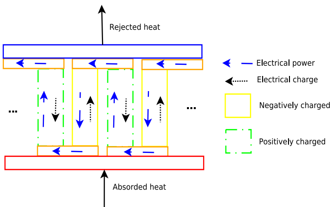
Fig. 1: ThermoElectric Generator (TEG)
