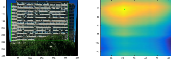
FIGURE 6 – Indice s_{cc} calculé pour toutes les positions (x, y) d'une fenêtre de taille (l, h) correspondant à la vérité terrain (en vert). La position (x, y) d'une fenêtre est celle de son coin supérieur gauche.
