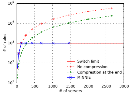
FIGURE 1: Simulation fat tree : nombre maximum de règles en fonction du nombre de serveurs.
