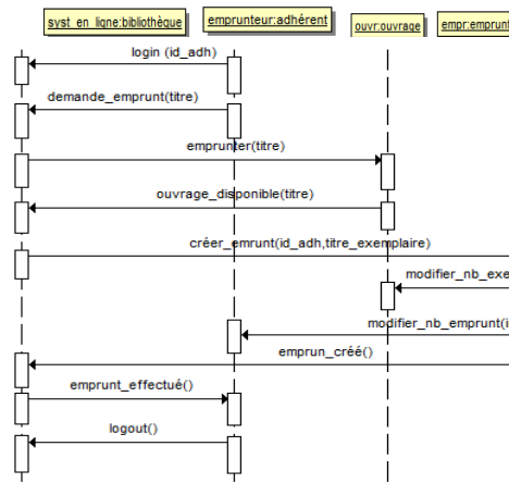
Figure 2. Diagramme de séquence du cas d'utilisation « emprunter »
