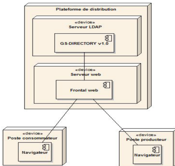
Figure 7. Architecture de déploiement des composants de test
