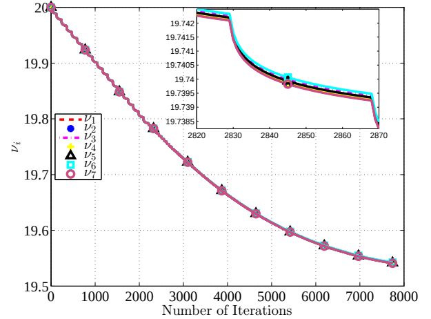
Fig. 4: Lagrange prices \nu_i
