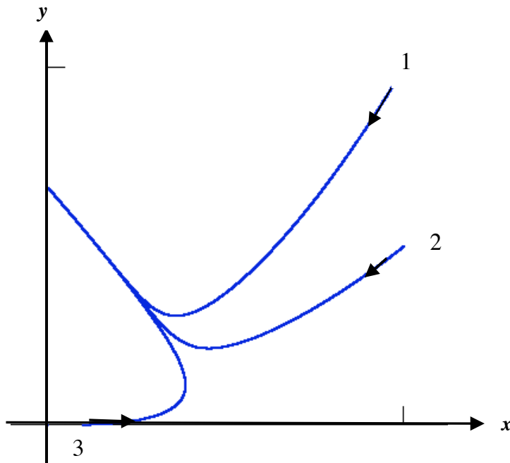
Figure 3. Portrait de phase d'une équation de compétition de Volterra
