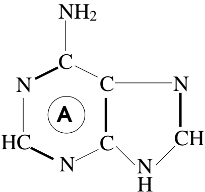
Adénine
