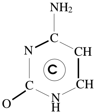
Cytosine
