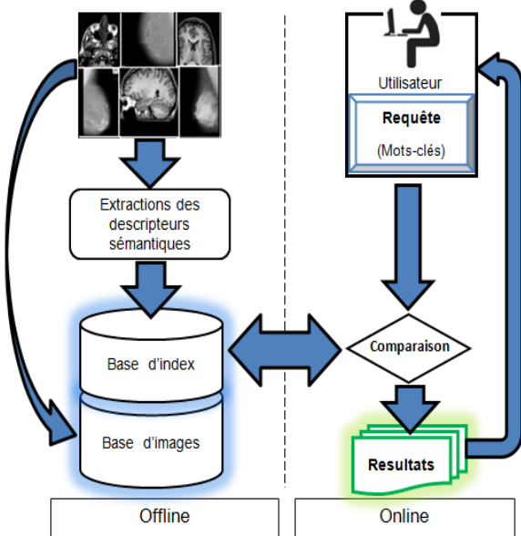
Fig.1 Architecture typique d'un système d'indexation d'images par les descripteurs sémantiques.
