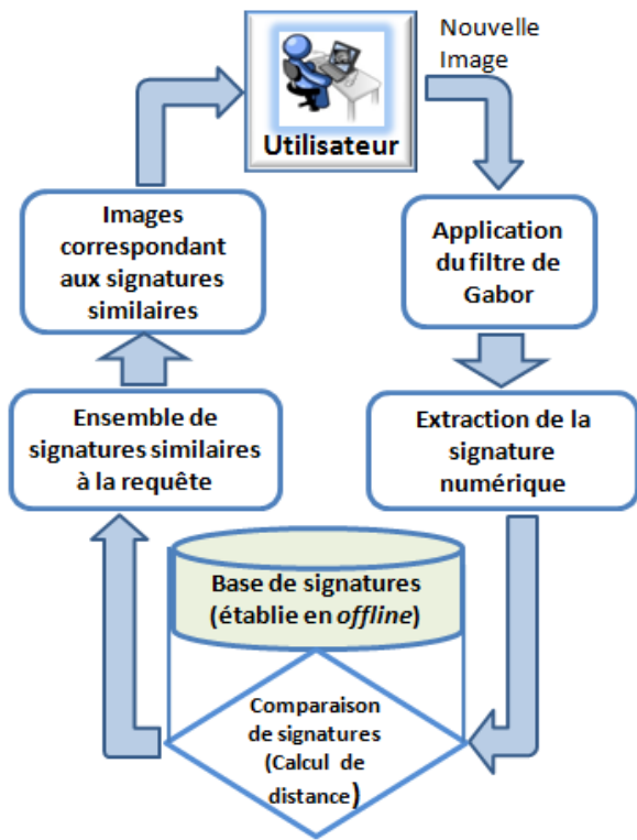
Fig.5 Principales étapes de la recherche par le contenu des images indexées par l'ondelette de Gabor
