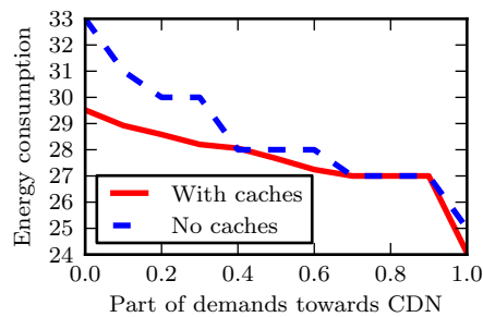
(b) Nobel-EU
