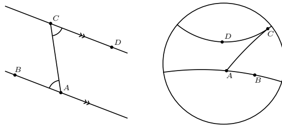
FIGURE 6 – Le postulat des angles alternes-internes.
