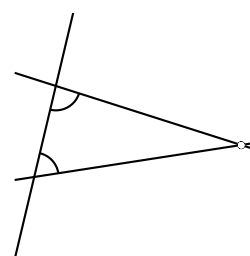
FIGURE 1 – Le 5 e postulat d'Euclide.
