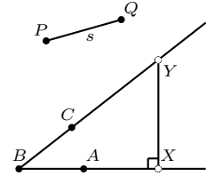
FIGURE 2 – Le postulat d'Aristote.
