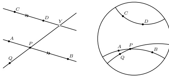
FIGURE 7 – Le postulat de Proclus.
