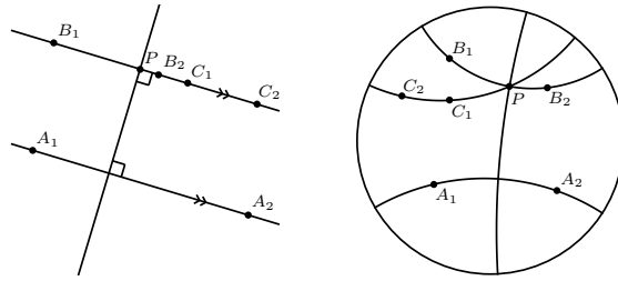
FIGURE 5 – Le postulat alternatif de Playfair.
