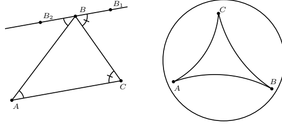
FIGURE 8 – Le postulat du triangle.
