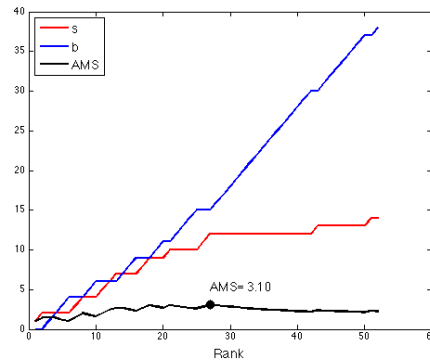
(d) AMS for radial
