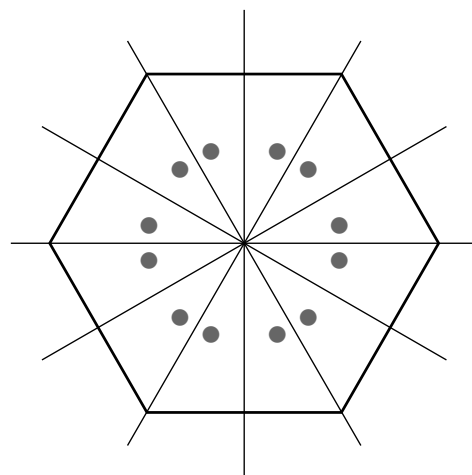
(d) Orbits with 2m=12 nodes
