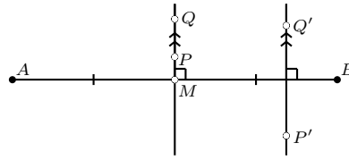
Fig. 56: Figure for lemma 36.
