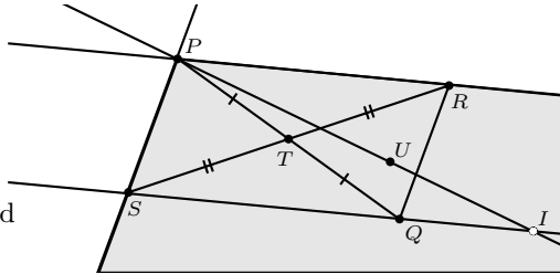
Fig. 49: Figure for lemma 32.
