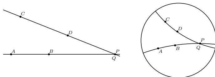
Fig. 18: Figure for lemma 3.
