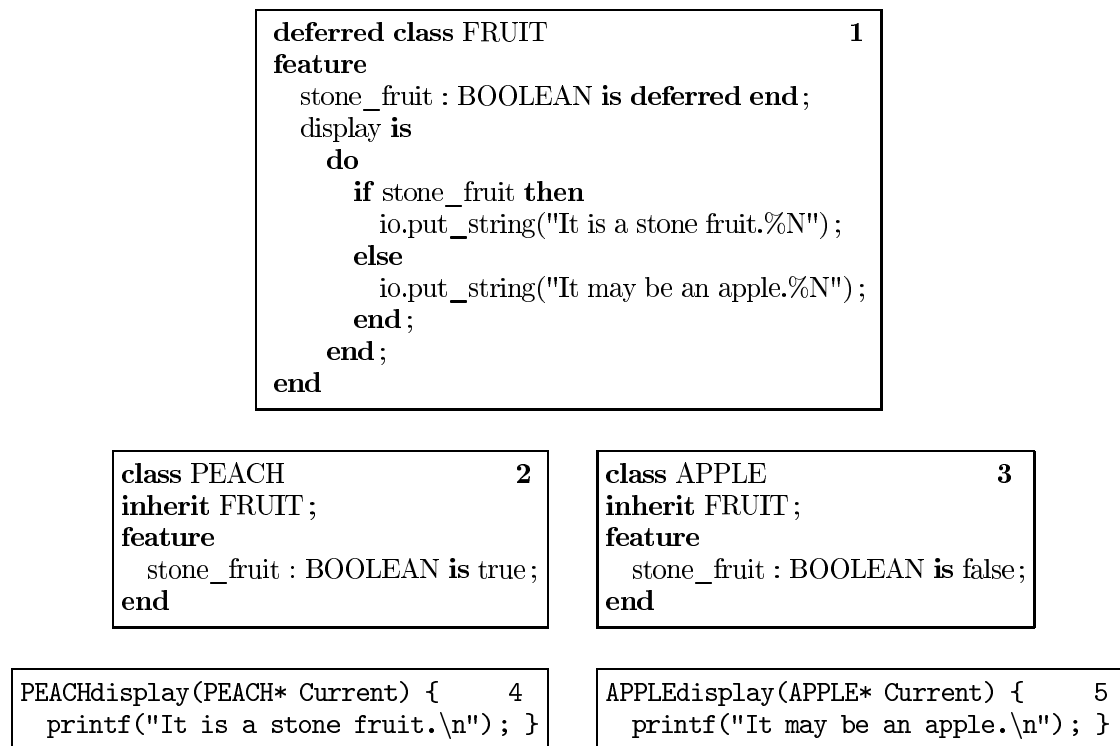
FIG. 1 – Spécialisation du code généré pour la méthode display définie dans la classe FRUIT . Les cadres 1 , 2 et 3 correspondent respectivement au source Eiffel des classes FRUIT , PEACH et APPLE . Les cadres 4 et 5 montrent le code C généré pour les classes PEACH et APPLE .
