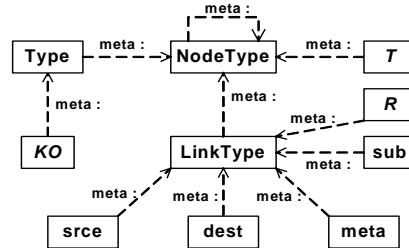
Figure 7. Éléments de base du méta-métamodèle M3
