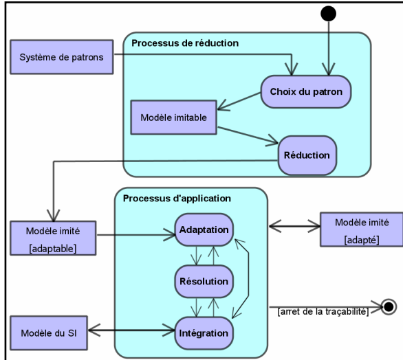
Figure 1. Processus d'imitation
