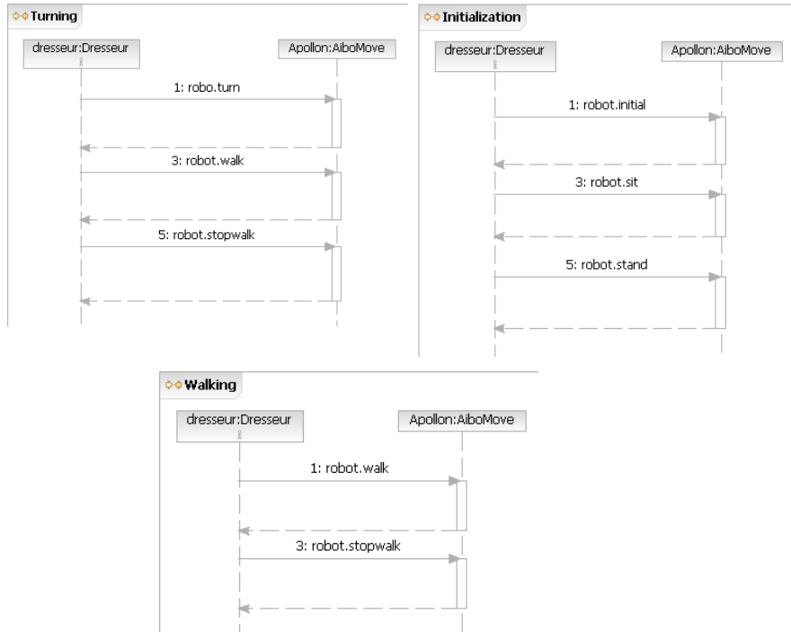
Figure 3 : Exemple de diagrammes de séquence de base pour AIBO
