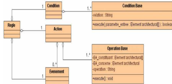
Figure 7: Modélisation d'une règle d'évolution
