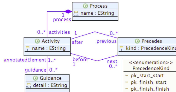
Figure 1. Le méta-modèle Ecore de SimplePDL
