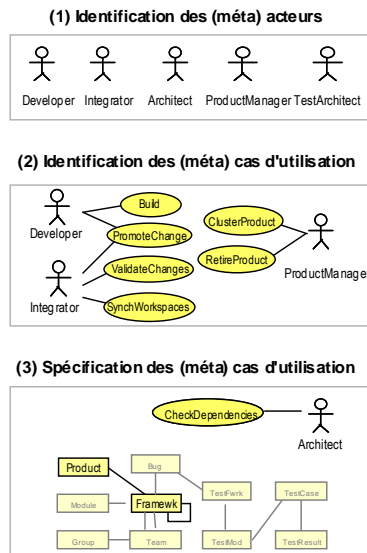
Figure 4. Meta-acteurs/Meta-besoins
