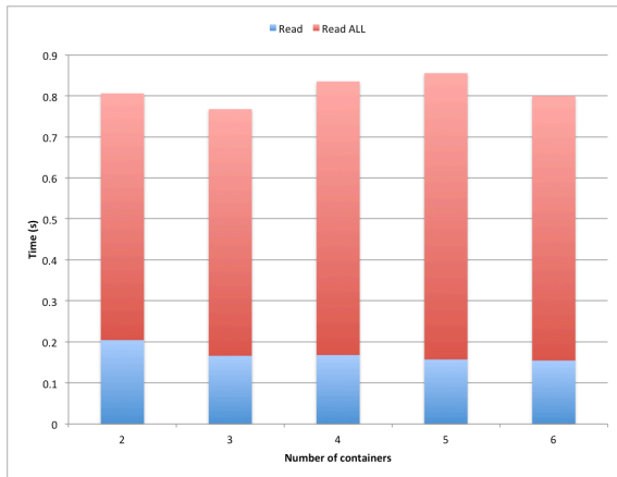
Figure 7.Évaluation d'une stratégie mixte HBase/Hive en fonction du nombre de conteneurs utilisés.
