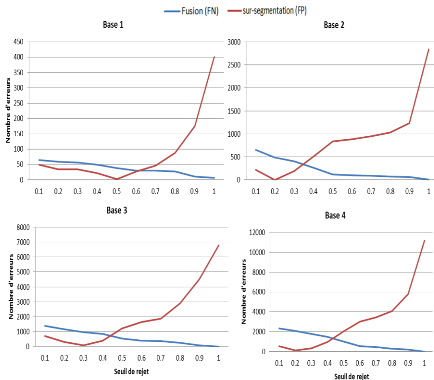
Figure 9. Relation entre le seuil et la fonction de rejet
