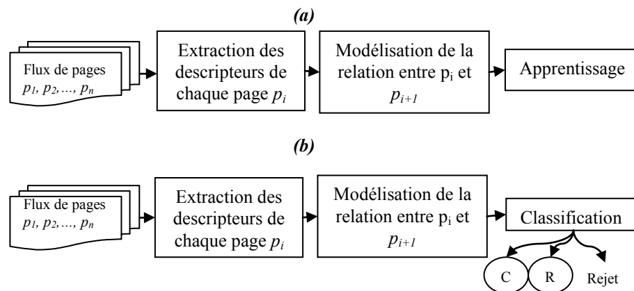
Figure 1. Organigramme de la segmentation de flux de documents, basée sur la classification supervisée : (a) apprentissage, (b) test
