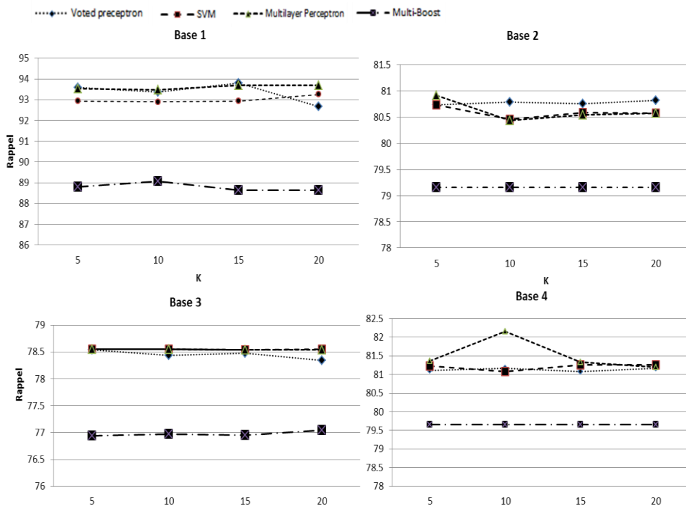
Figure 8. Evaluation de la relation R sur les 4 bases en utilisant 4 classifieurs
