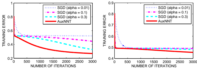
(a) 1 hidden layer autoencoder (b) 2 hidden layers autoencoder
