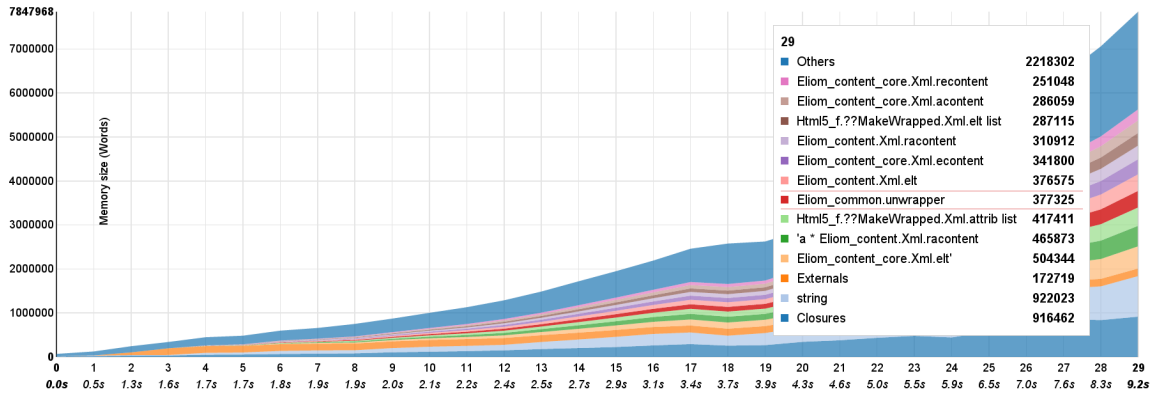
FIGURE 9 – Graphique mémoire généré à l'aide d'ocp-memprof sur une utilisation de l'application Cumulus.
