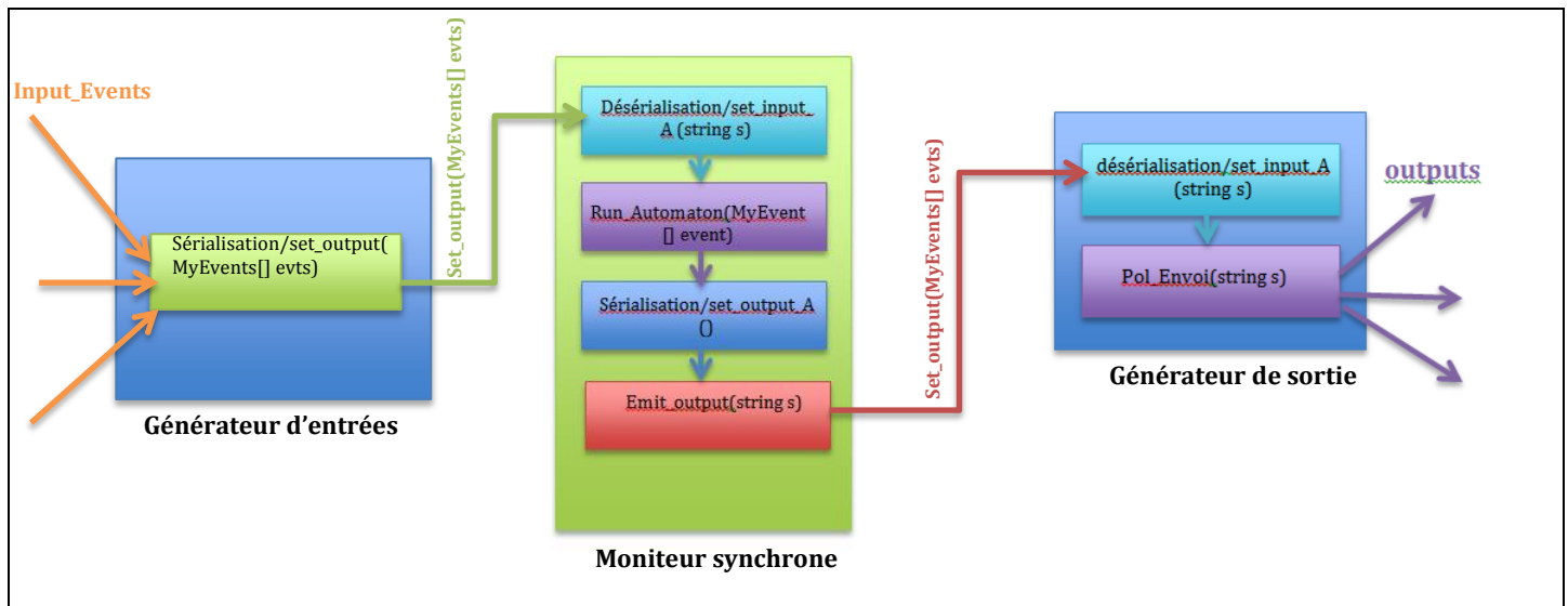
Figure 23: sérialisation/désérialisation : fonctionnement complet
