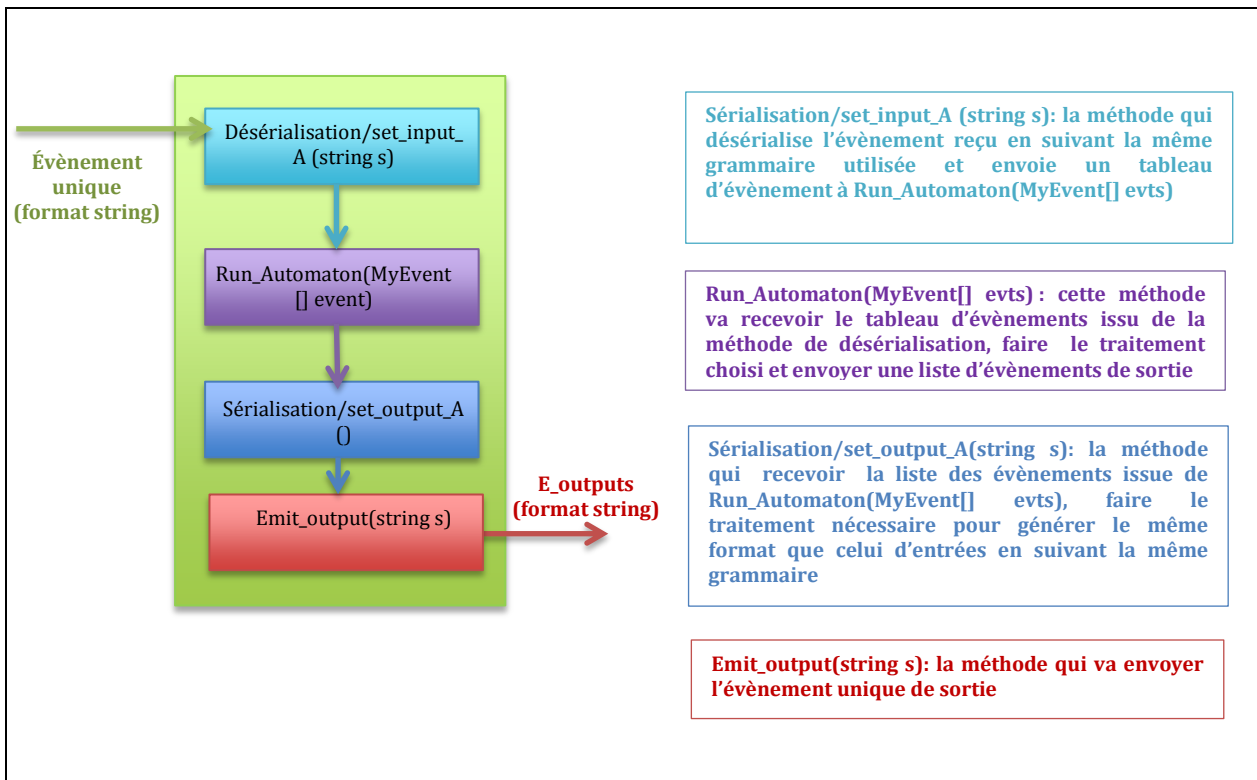
Figure 21 : utilisation de la sérialisation/désérialisation dans le moniteur synchrone
