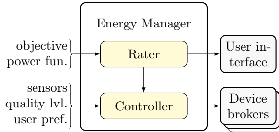
FIGURE 1 – Le composant gestionnaire énergétique.
