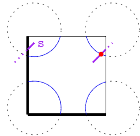
Fig. 2. Periodic oracle
