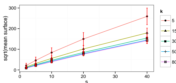
Figure 3. Surface moyenne des zones cohérentes en fonction de s . La courbe illustre la racine carrée de la surface en nombre de pixels.
