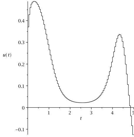
Fig. 2: Ornstein-Uhlenbeck (control)
