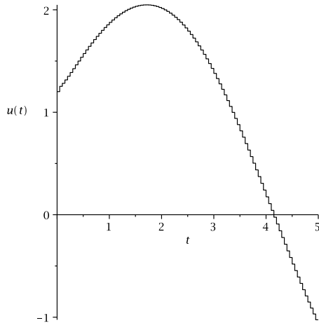
Fig. 4: Ornstein-Uhlenbeck (control)
