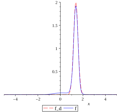
Fig. 5: Ornstein-Uhlenbeck
