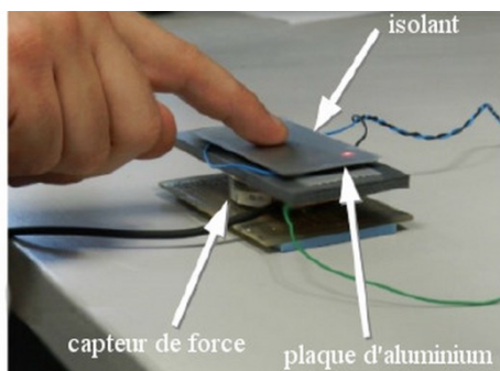
Fig. 6 Dispositif expérimental utilisé
