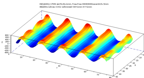
Fig. 3 : Cartographie du mode de vibration recherché ( f_r = 38220 Hz)
