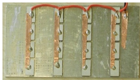
Fig. 4 Disposition des céramiques piézoélectriques collées sur la face inférieure de la plaque à mettre en vibration
