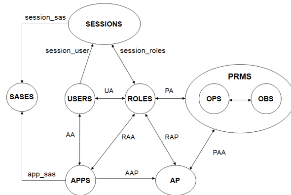
Fig. 1. Core RBAC^+
