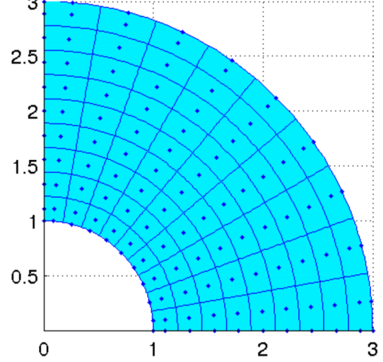
(d) Interpolation grid (Greville nodes) for the IIL method, 121 nodes.
