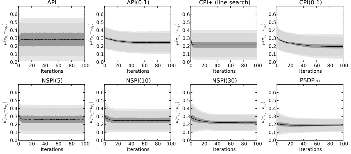
FIGURE 2 – Statistiques pour toutes les instances. Les PDMs (M_i)_{1 \leq i \leq 30} sont i.i.d. et ont la même distribution que M_1 . Conditionnellement à un PDM M_i et un algorithme, les mesures d’erreur pour toutes les itérations k sont i.i.d. et ont la même distribution que L_{1,k} . La ligne centrale des courbes d’apprentissage donne un estimé empirique de la moyenne globale (\mathbb{E}[L_{1,k}])_k . Les trois régions grisées (du plus foncé au plus clair) sont respectivement des estimés de la variabilité (sur les PDMs) (\mathbb{E}[\text{Std}[L_{1,k}|M_1]])_k de l’erreur moyenne, la moyenne (sur les PDMs) (\mathbb{E}[\text{Std}[L_{1,k}|M_1]])_k de la déviation standard de l’erreur, et la variabilité (sur les PDMs) (\text{Std}[\text{Std}[L_{1,k}|M_1]])_k de la déviation standard de l’erreur. Pour faciliter les comparaisons, toutes les courbes sont affichés avec les mêmes axes x et y .
