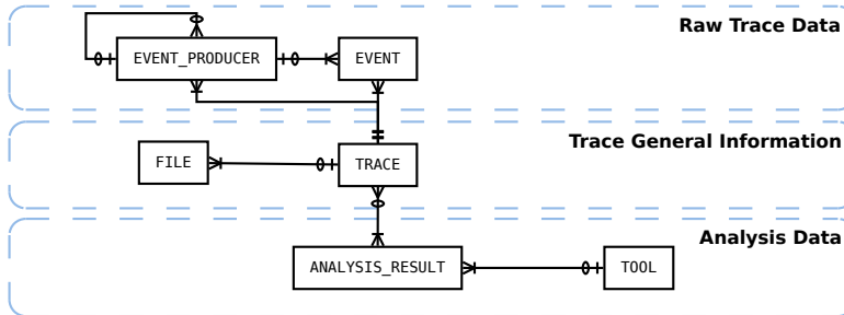
FIGURE 2 – Modèle de données dans FrameSoC.
