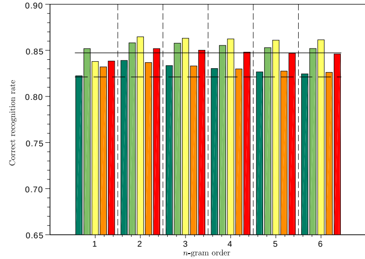
(d) S = 20 , Witten-Bell smoothing
